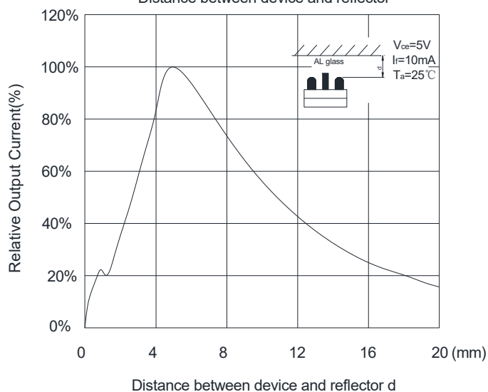
相对输出电流VS器件与反射器之间的距离曲线图
