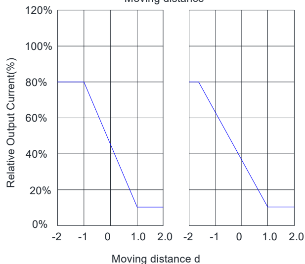
相对输出电流VS器件与移动距离曲线图
